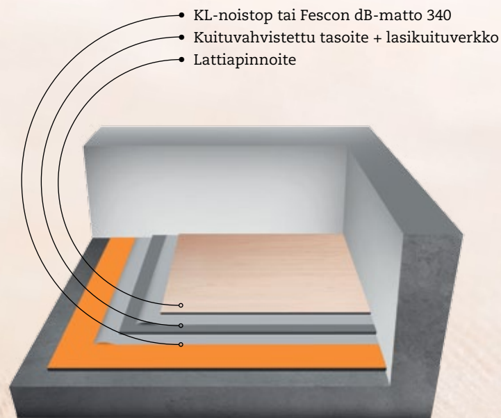
Fescon dB-lattian rakenne
