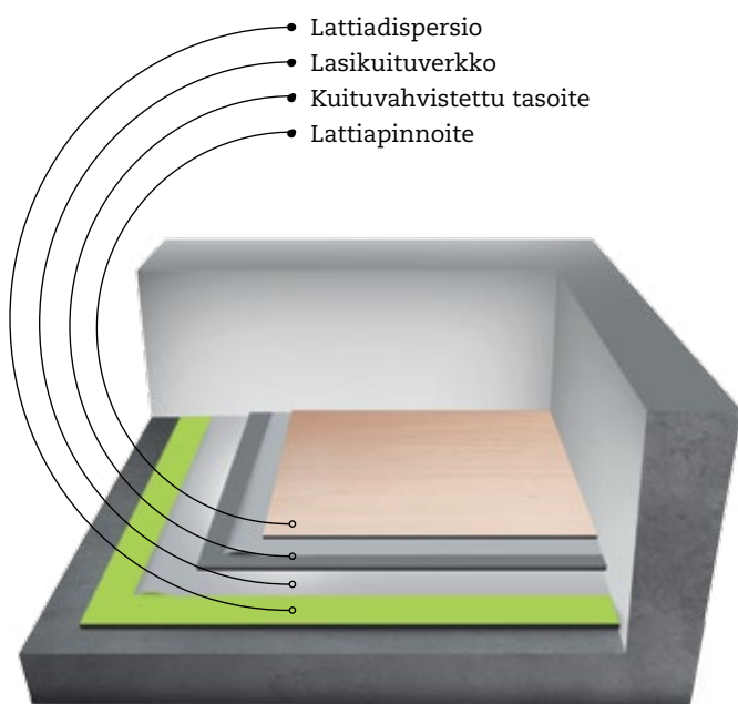
Fescon korjauslattian rakenne
