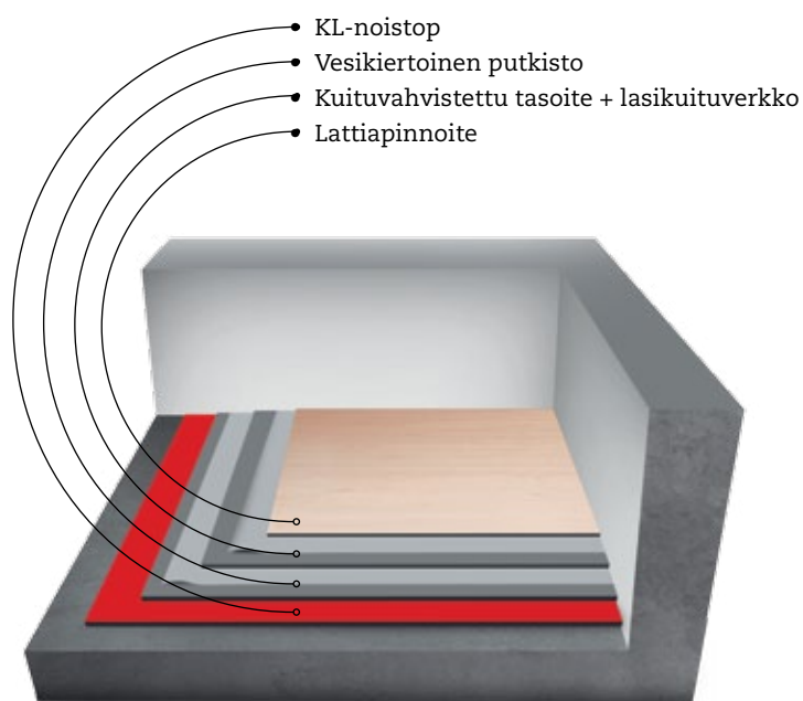
Fescon lämpölattian rakenne
