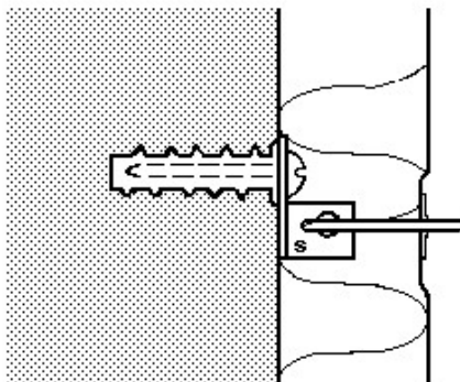
Heilurihaka lukitusasennossa ja villa asennettuna
