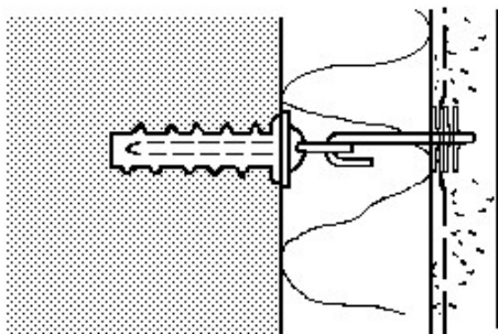
Lopputilanne halkaistuna ylhäältä päin katsottuna
