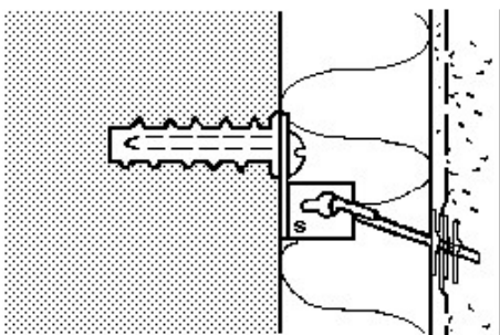
Sivukuva halkaistuna lukituslevyt asennettuna ja rapattuna
